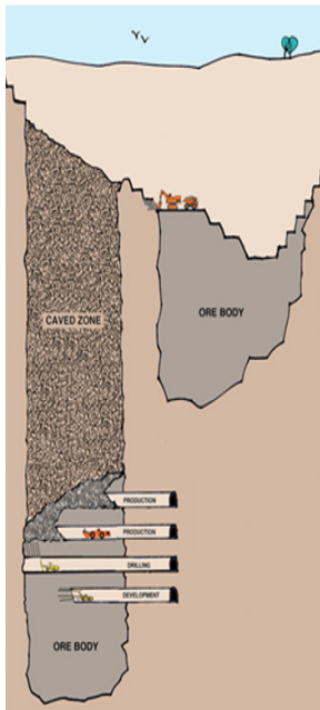
Sublevel Caving
