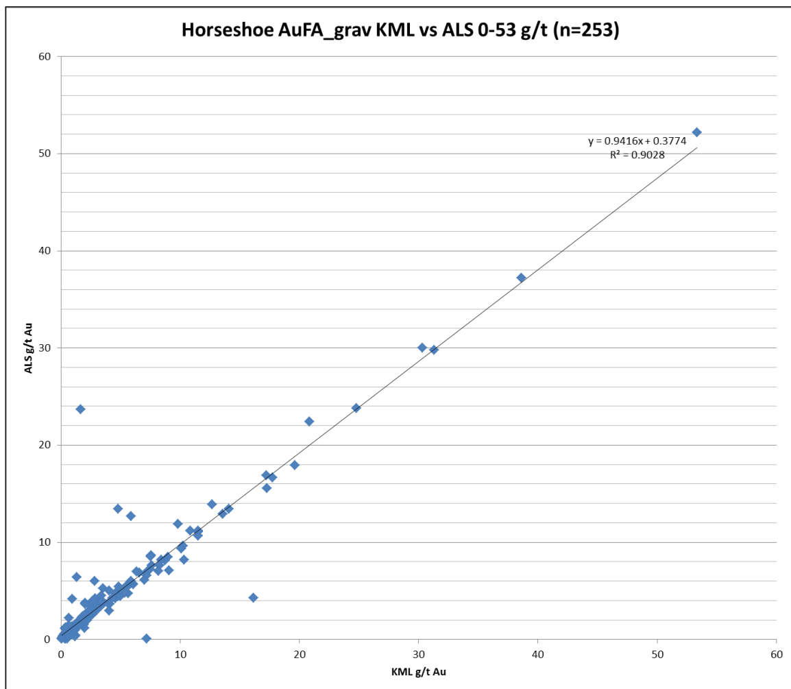
Figure 12-2: Horseshoe AuFA_grav KML vs. ALS 0-53 g/t (n=253)
