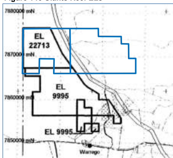
Figure 146 Giants Reef ELs
