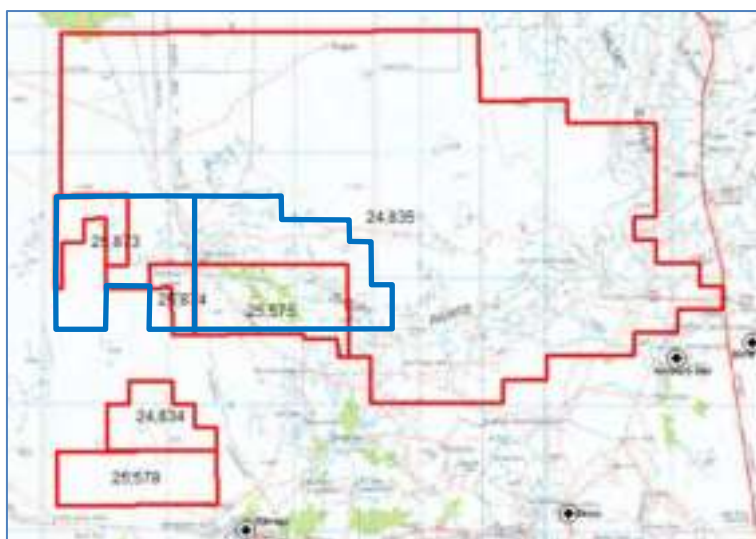
Figure 158 Uranium West / Rum Jungle ELs
