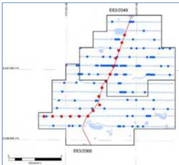
Figure 52 AngloGold auger holes in eMetals ELs
