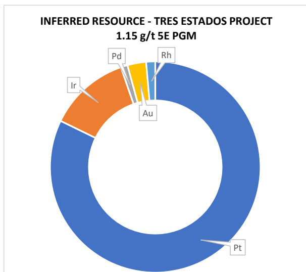
Figure 3: Inferred 5E PGM Resource (relative grade), Três Estados
