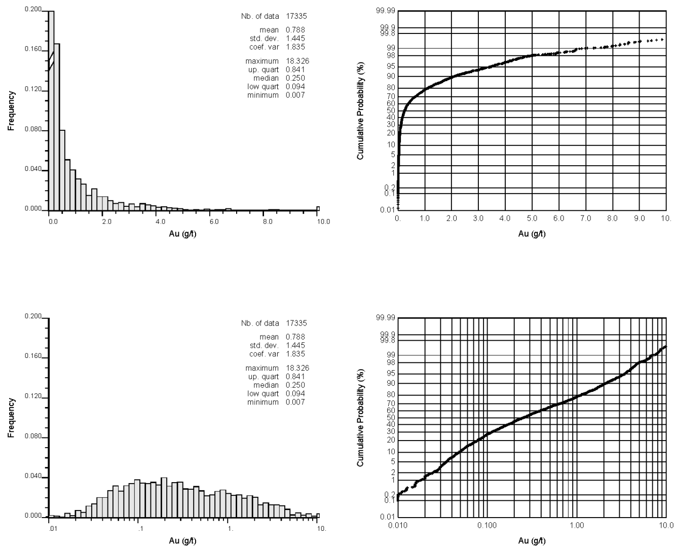
Figure 12-3 Histogram of 10m ALS Composites
